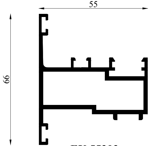
EX 55303 1.223 KG/M IX= 8.68 CM 4 IY= 17.85 CM 4
