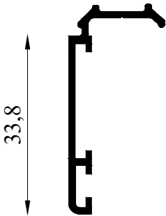
DW 12303 0.235 KG/M IX= 1.55 CM4 IY= 0.20 CM4
