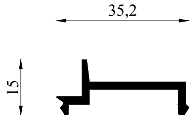
EX 55304 0.279 KG/M IX= 0.08 CM 4 IY= 1.27 CM 4
