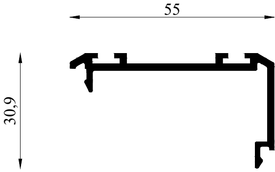
EX 55302 0.510 KG/M IX= 1.11 CM 4 IY= 6.75 CM 4
