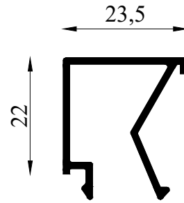
EX 55401 0.284 KG/M IX= 0.84 CM4 IY= 0.62 CM4
