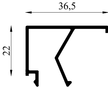
EX 55400 0.324 KG/M IX= 0.98 CM4 IY= 1.27 CM4
