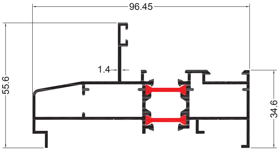
TV 4302 1.481 Kg/m.
