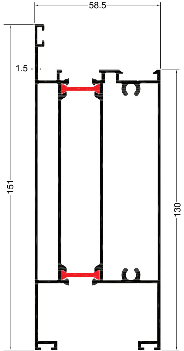
TV 4301 2.686 KG/M
