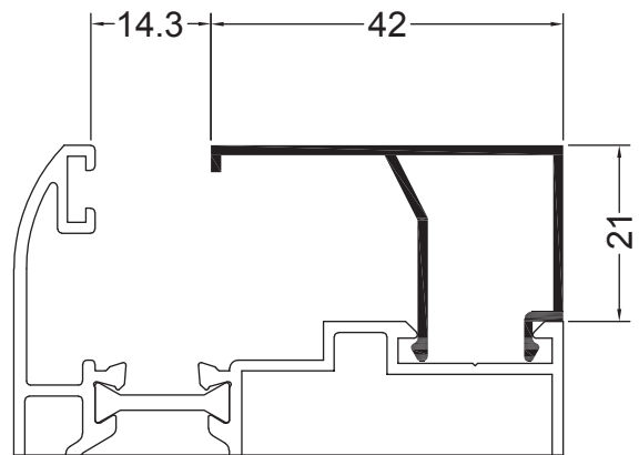
TV 4401 0.335 KG/M
