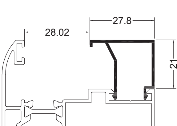
TV 4400 0.273 KG/M
